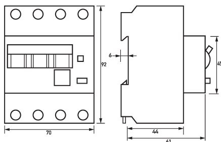
Maßzeichnung FI-/LS-Kombinationen DRCBO 4 B16/0,03/3N-A
