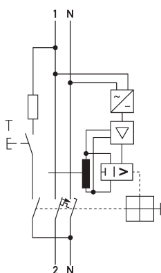
Schaltungsbeispiel FI-/LS-Kombinationen DRCBO 4 B16/0,30/1N-B SK
