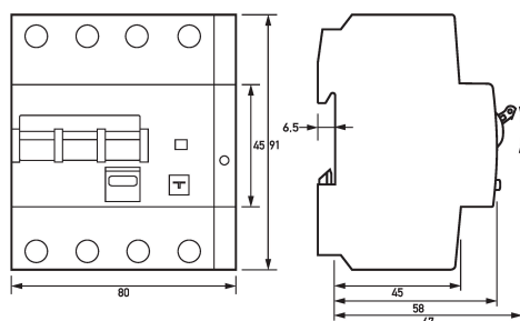
Maßzeichnung FI-/LS-Kombinationen DRCBO 4 C16/0,03/3N-B SK
