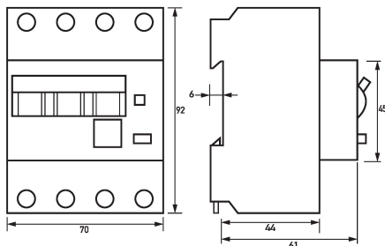
Maßzeichnung FI-/LS-Kombinationen DRCBO 4 C32/0,03/3N-A
