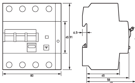
Maßzeichnung FI-/LS-Kombinationen DRCBO 4 C32/0,03/3N-B SK
