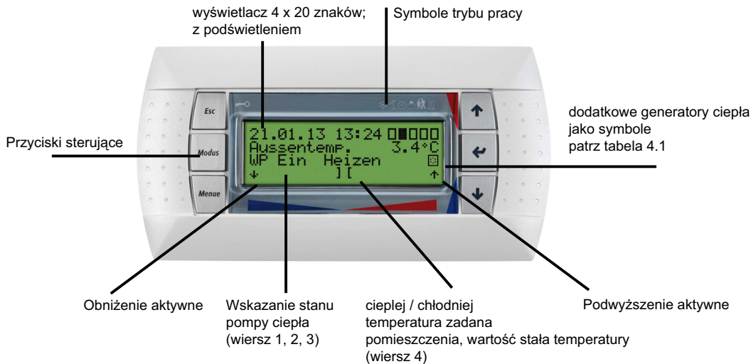
Rys. 4.1: Sterownik pompy ciepła z oddzielnym standardowym wyświetlaczem LCD z przyciskami do obsługi
