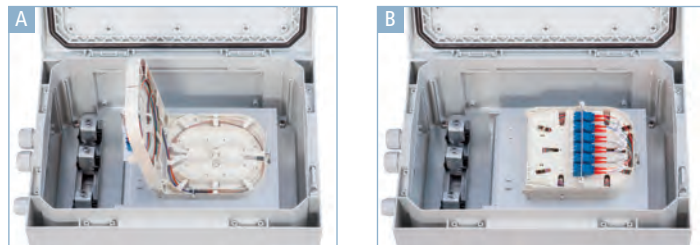
Klappbare Spleißkassette zur leichten Montage
