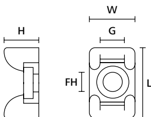
Befestigungssockel KR- und CTM-Serie
