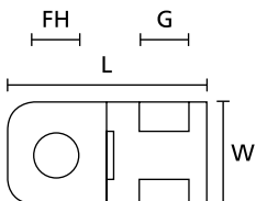
Befestigungssockel CTAM-Serie
