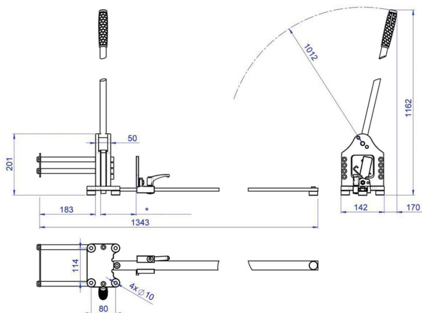
Kuva 2: Mitat mm
