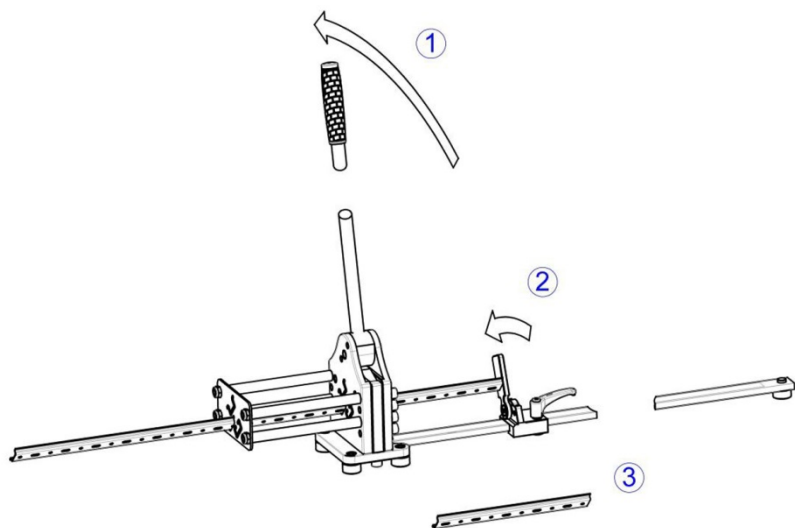
Kuva 8: Kannatinkiskon poistaminen
