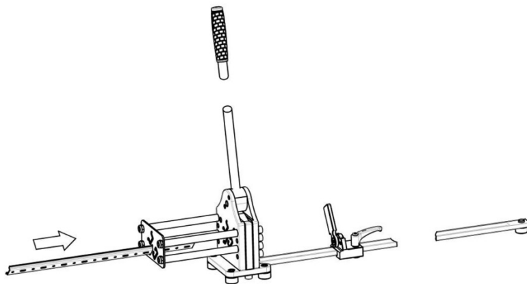
Kuva 6: Kannatinkiskon sisääntyöntäminen
