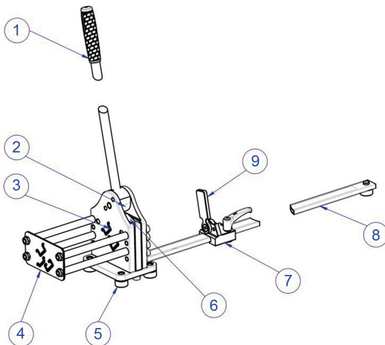
Kuva 1: Kokonaisnäkömä
