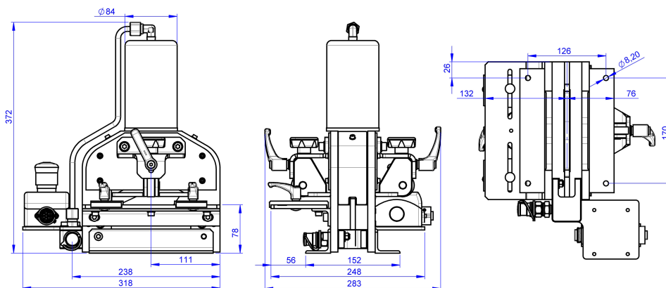
Εικ. 2: Διαστάσεις
