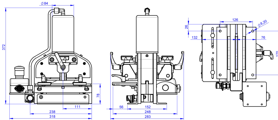
Imagen 2: Dimensiones
