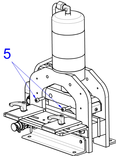
Imagen 7: Extraer los tornillos de fijación
