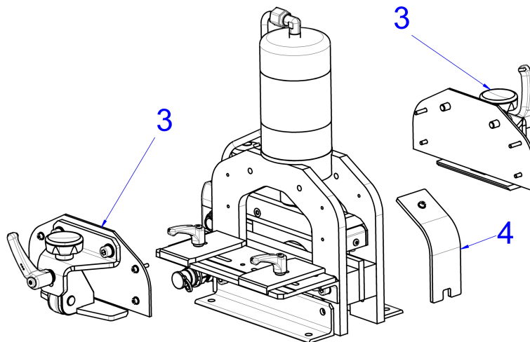
Rys. 11: Demontaż dociskaczy
