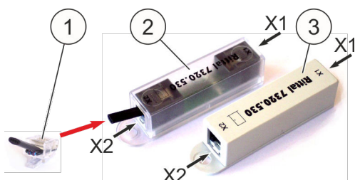
Fig. 49: Contattore anta e resistenza terminale (RJ12)
