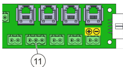
Fig. 10: Attacco per monitoraggio e comando di serbatoio esterno
