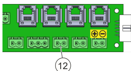
Fig. 11: Attacco rilevatore portatile
