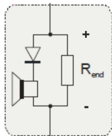
Fig. 45: Schema dei collegamenti elettrici
