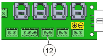
Fig. 38: Attacco rilevatore portatile
