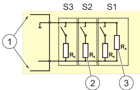
Fig. 55: Rilevatore portatile collegato in parallelo
