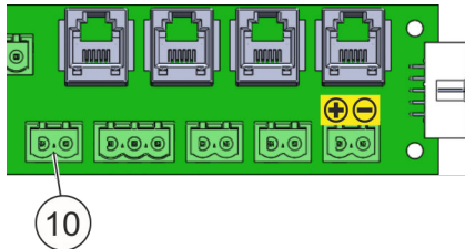
Fig. 44: Attacco per dispositivo d'allarme esterno
