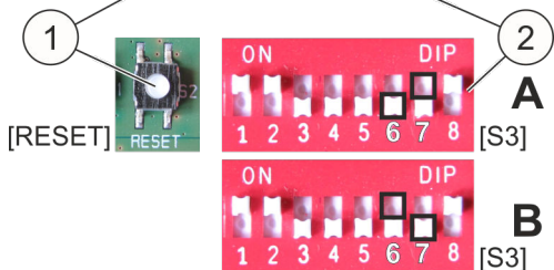
Fig. 50: [Tasto Reset] e DIP switch "S3"
