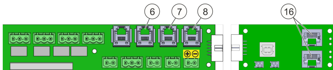
Fig. 46: Attacchi CMC
