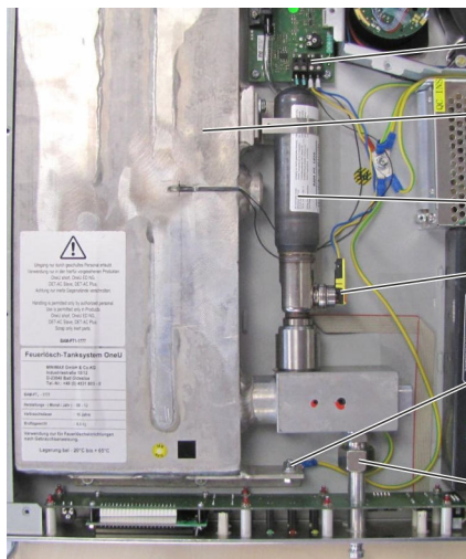
Fig. 80: Vista d'insieme del serbatoio
