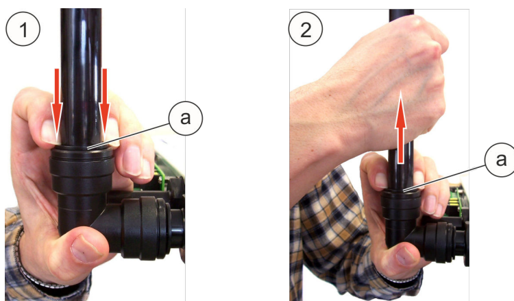
Fig. 32: Smontaggio
