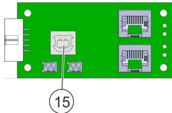
Fig. 13: Porta USB (tipo B)
