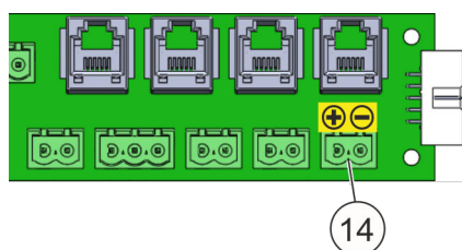
Fig. 12: Alimentazione di tensione
