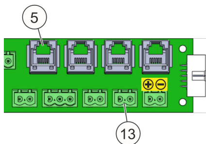
Fig. 7: Attacchi per contattore anta
