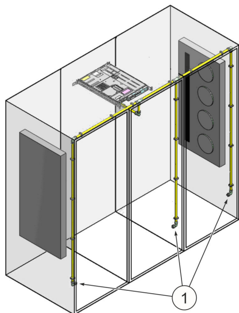
Fig. 33: Monitoraggio di più armadi
