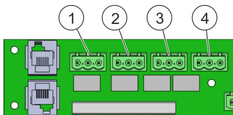
Fig. 6: Uscite relè
