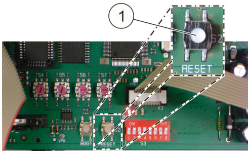
Fig. 73: [Tasto Reset]
