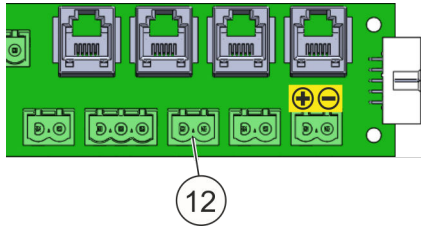
Fig. 54: Morsetto di collegamento "Rilevatore portatile"
