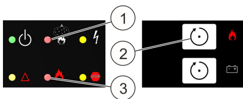
Fig. 41: LED e tasto [Reset]
