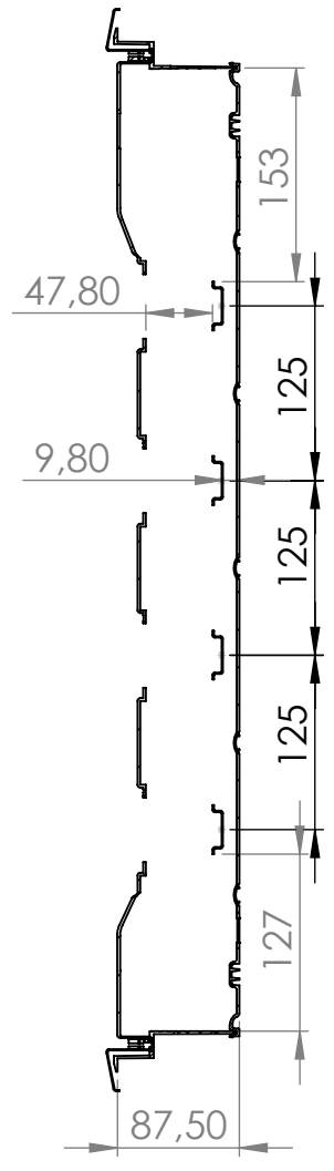
B-B (1 : 6)
