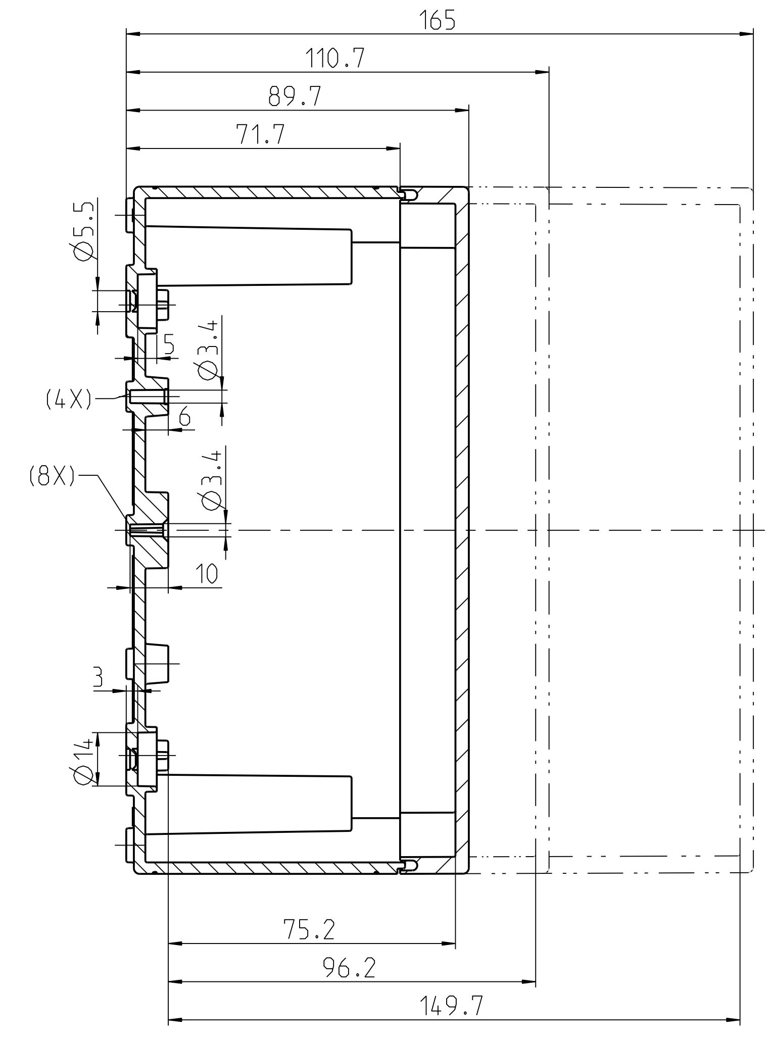
A-A
