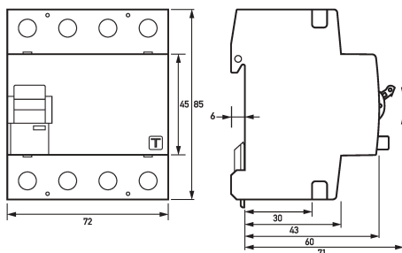
Maßzeichnung Fehlerstromschutzschalter DFS 4 040-4/0,30-B SK ISO HD
