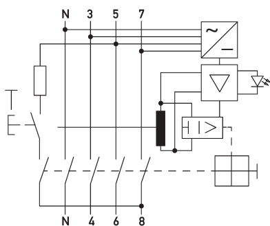
Schaltungsbeispiel Fehlerstromschutzschalter DFS 4 040-4/0,30-B SK ISO HD
