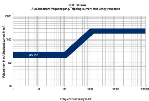
Diagramme Fehlerstromschutzschalter DFS 4 040-4/0,30-B SK ISO HD
