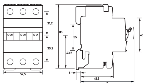
Maßzeichnung Gruppenansicht
