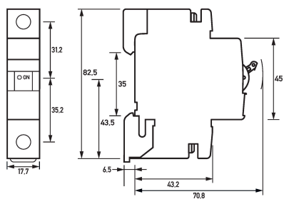
Maßzeichnung Leitungsschutzschalter DLS 6hdc B4-1
