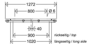
Zusätzliche Kabeleinführungen rückseitig (mit Presshaut) Additional entries (knock-outs)
