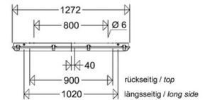
Zusätzliche Kabeleinführungen rückseitig (mit Presshaut) Additional entries (knock-outs)
