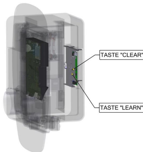
Abbildung 4 Bedienfeld des RFID-Moduls
