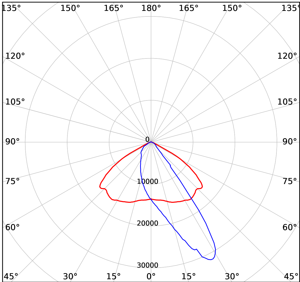
cd 40000 lm — C0-C180 — C90-C270
