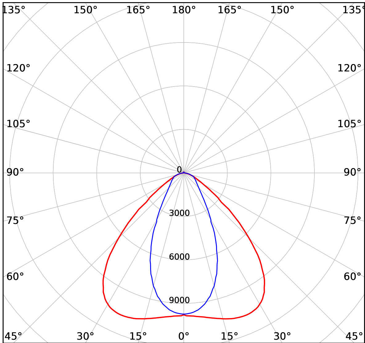
cd — C0-C180 — C90-C270 16000 lm
