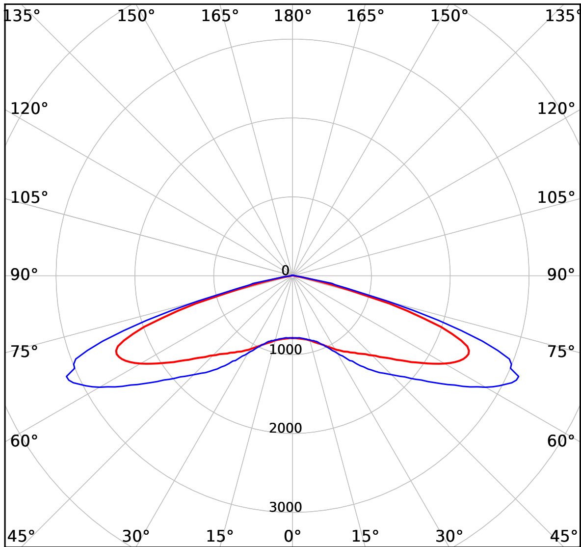
cd 8800 lm — C0-C180 — C90-C270
