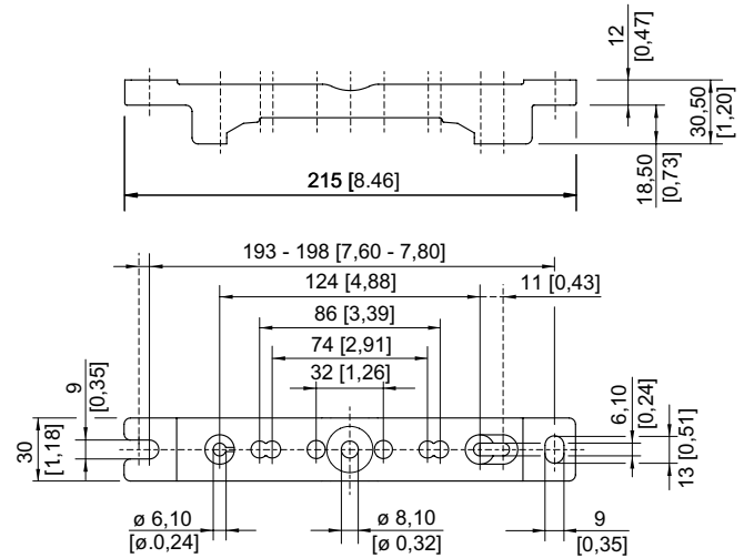
Montageschiene
