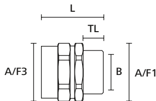
HelaGuard Verschraubung, gerade mit starrem Außengewinde
