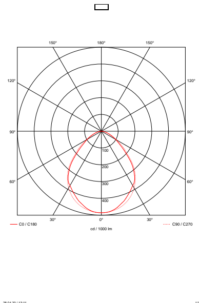
LumE® PRACHT_BERNINA_F_Idt_1x32W_breit90_1274mm.Idt. ©Pracht Diagram
