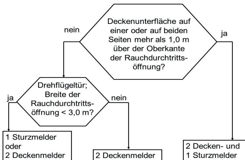
Bild 3: Entscheidungsdiagramm
