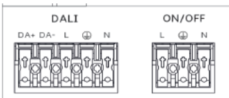
Abb.: 4 Anschlusschema: Dali oder schaltbar
