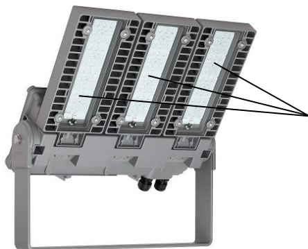
LED-Modulgehäuse mit eingebautem LED-Modul und Abdeckglas
