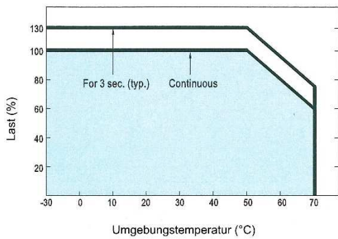
Temperatur/Ausgangsleistung
