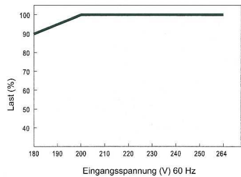
Eingangsspannung/Ausgangsleistung
