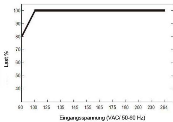
Eingangsspannung/Ausgangsleistung
