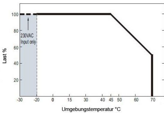
Temperatur/Ausgangsleistung
