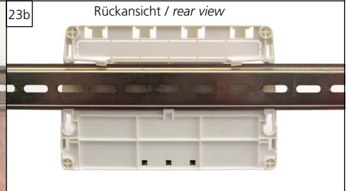
Rückansicht / rear view
