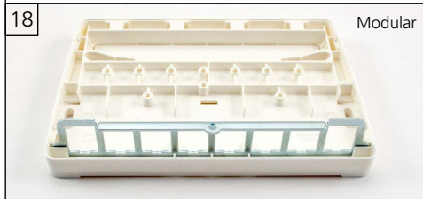
Einbau eines Moduls / Kupplung installation of Module / Coupler
