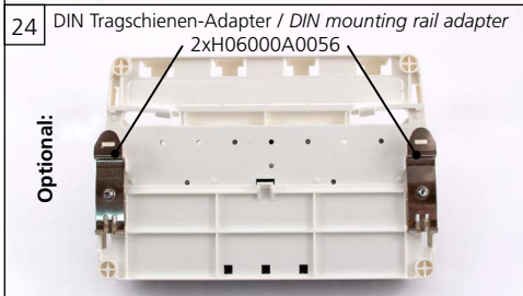
Für Tragschiene TH35 for mounting rail TH35 nach / acc. to DIN 60175
