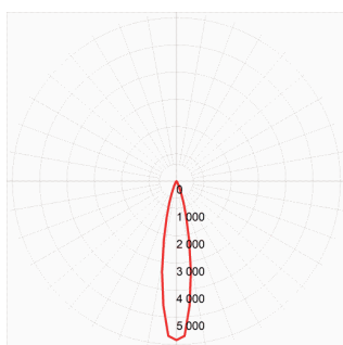
TLM1-18°
