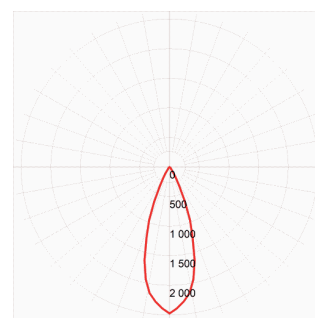
TLM1-36°
