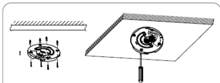
Abb. 3 Montageplatte befestigen
