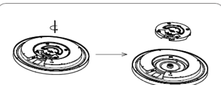
Abb. 7 Leuchte und Montageplatte trennen
