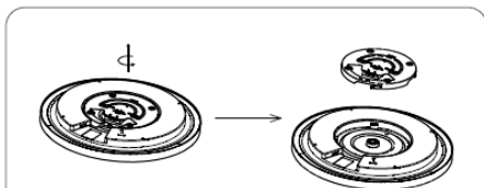
Abb. 1 Leuchte und Montageplatte trennen
